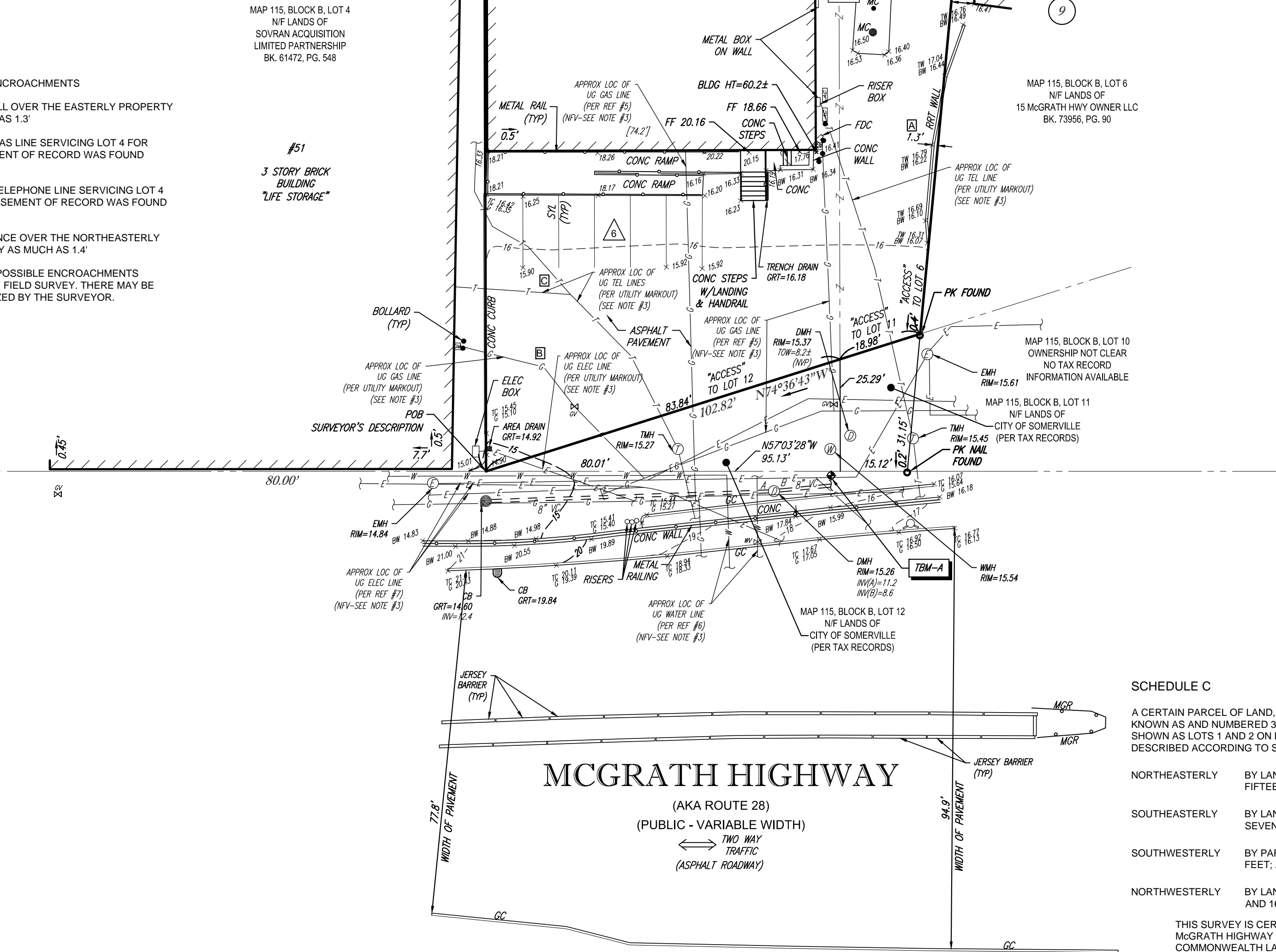
DETAIL SCALE: 1" = 10'
