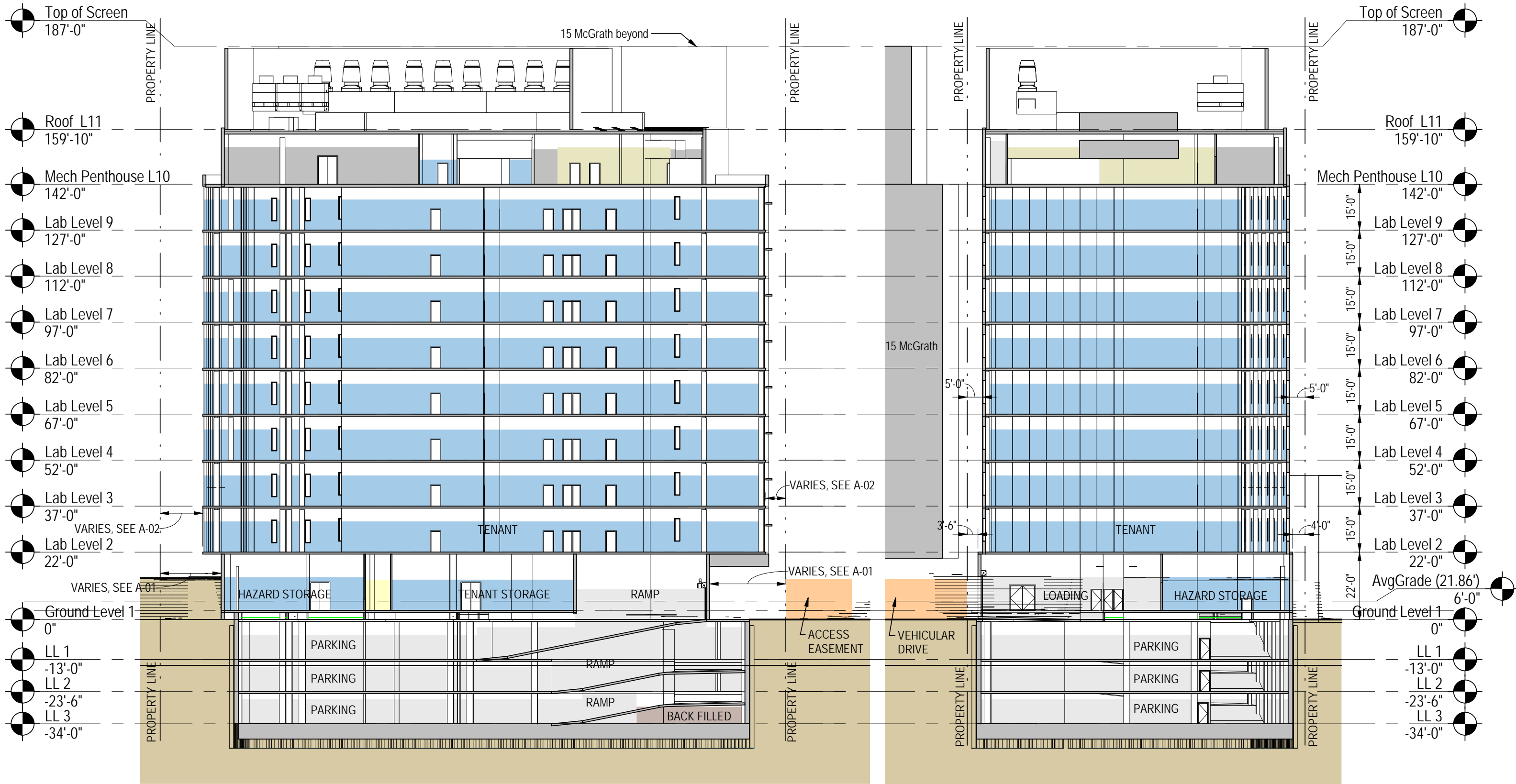
LONGITUDINAL SECTION THRU RAMP
